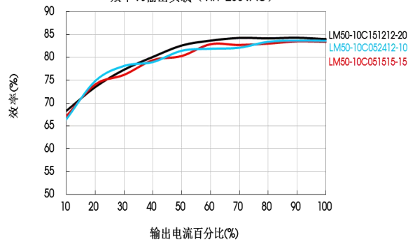
效率Vs输出负载 (Vin=230VAC)
